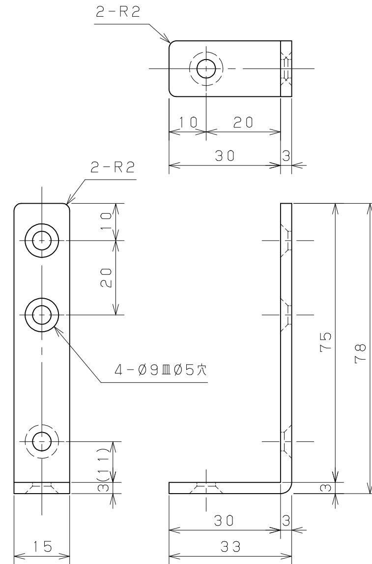
7 上がり框固定金具 (小) S=1/1
